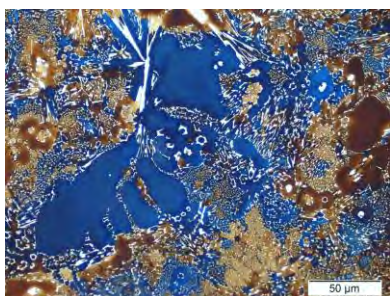
« Papillon bleu » Composite à matrice métallique renforcé par des particules de céramique - Valérie Daeschler - Arcelor Mittal
