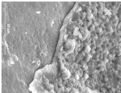
« Ressac » - Oxyde écaillé sur acier K41X Maria Rosa Ardigo-Besnard - Laboratoire ICB
