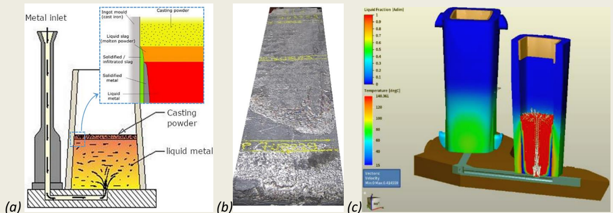
Coulée de lingots en source et sa modélisation : (a) schéma de la coulée en lingotière en source avec agrandissement sur la région où les différents domaines d'intérêt sont en contact, (b) surface d'un lingot d'acier inoxydable de longueur 1,4 m coulé avec des poudres à faible teneur en carbone, (c) prédiction logicielle du procédé de coulée industrielle d'un lingot de 4,2 tonnes.
