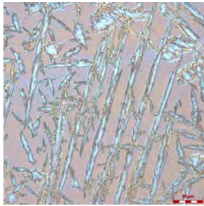
"Givre métallique" (Djan Koçak -DCNS) Acier inox duplex réalisé par fabrication additive
