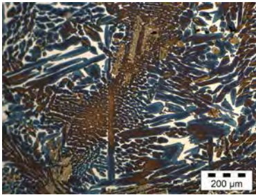
"Automne en acier" (Coralie Jung – ArcelorMittal) Attaque Nital sur acier type Lean Maraging
